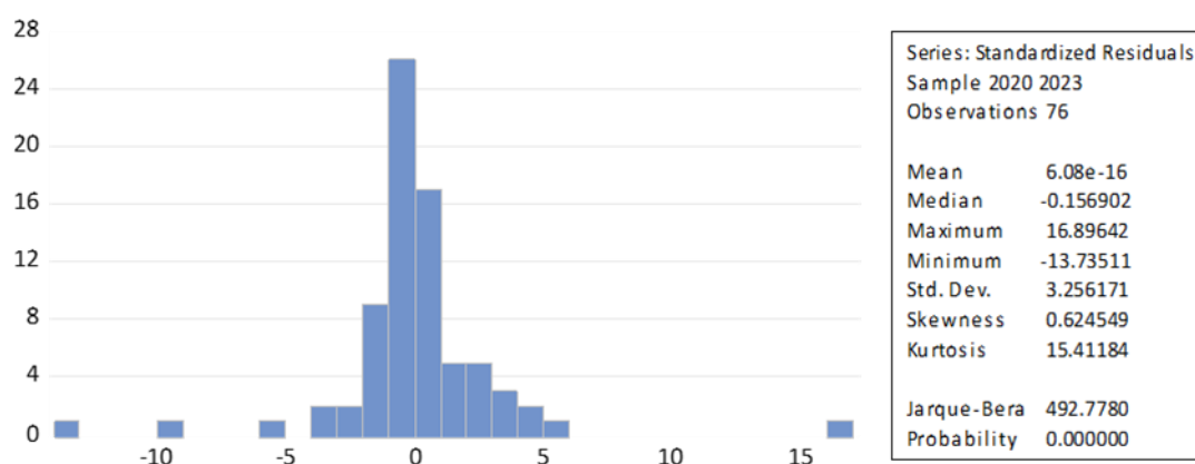
Gambar 1. Uji Normalitas
